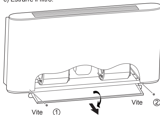
Figura 4-1 Diagramma della rimozione del filtro
