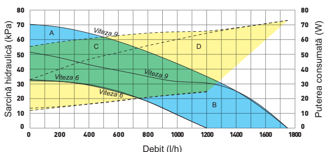
Grafic debit/sarcină hidraulică VICTRIX TERA V2 38 EU/ VICTRIX TERA V2 35 PLUS EU
