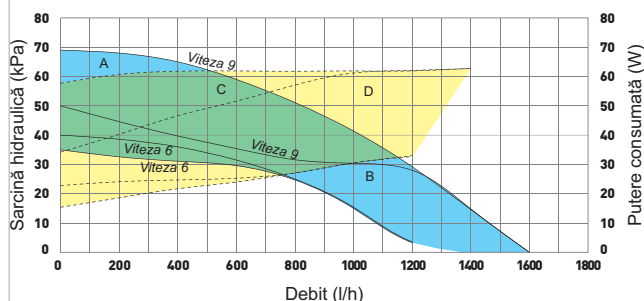
Grafic debit/sarcină hidraulică VICTRIX TERA V2 32 EU
