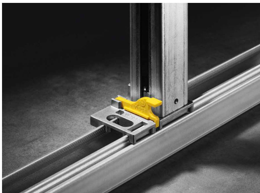
Prevista Dry Plus-Montare în șină: Piciorul este așezat simplu și înclichetat fix.
